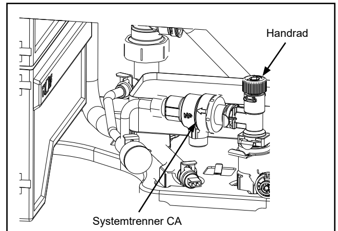
Bild: Befülleinrichtung als Nachrüstungsset im Gerät integrierbar
