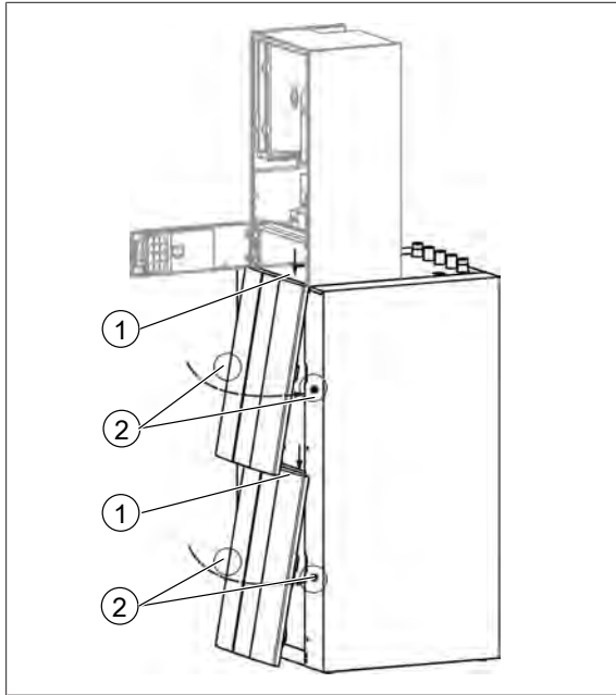
1 Einhängempunkte 2 Einrastpunkte
