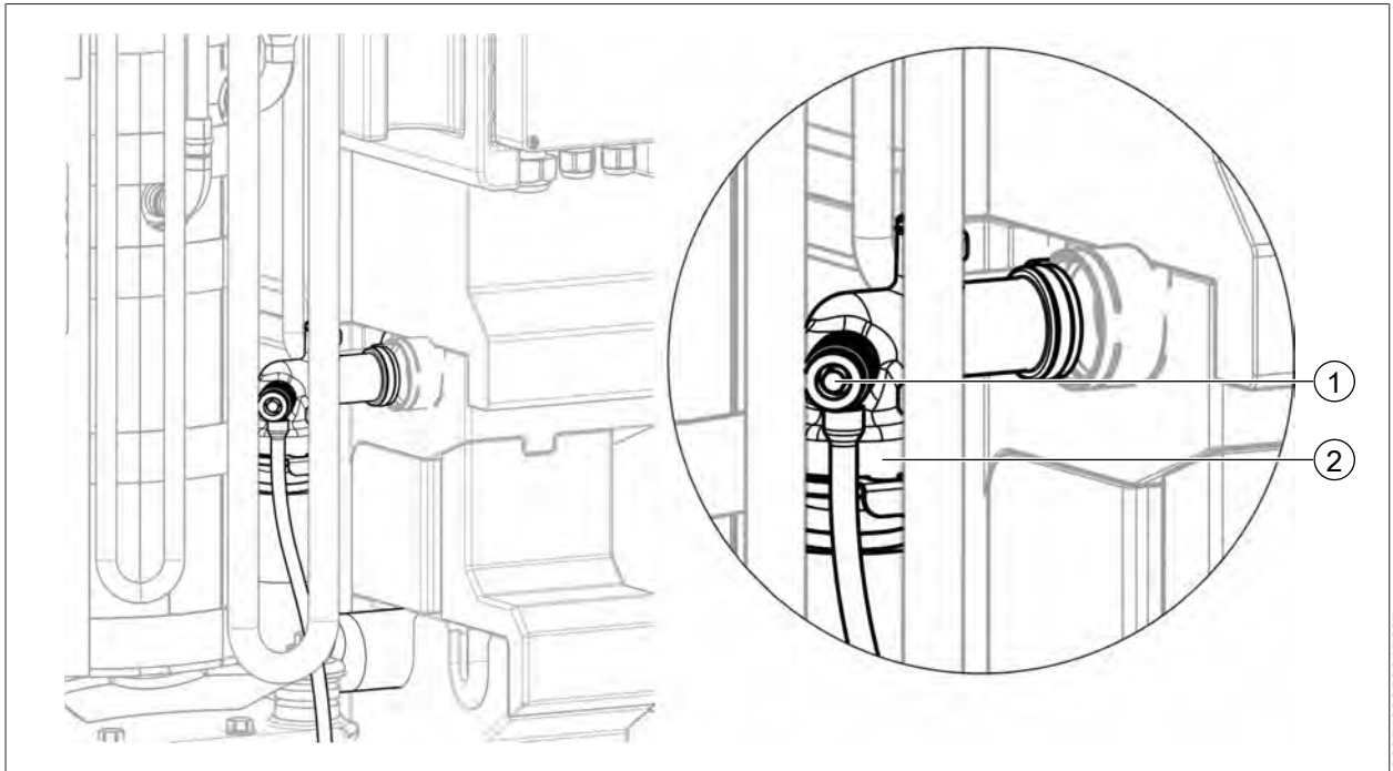
1 Entleerungshahn
