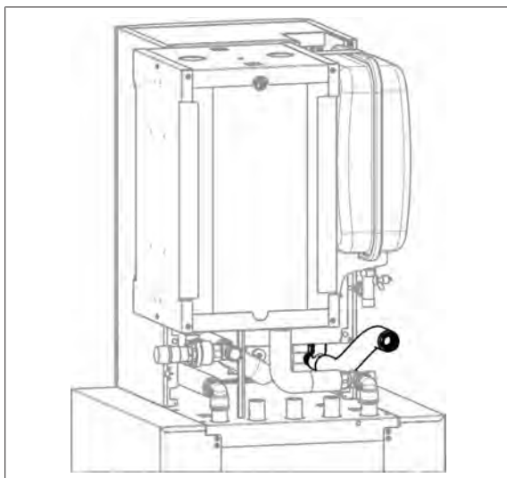
39. Vormontiertes Wellrohr (siehe Schritt 26) mit dem Anschlusswinkel in die Inneneinheit stecken und mit Verrohrungsclip DN 28 (Pos. 5.10) sichern.
