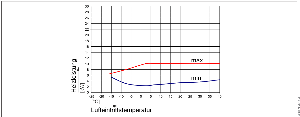
Abb. 8: Heizleistung CHA-10 bei einem Vorlauf von 65°C
