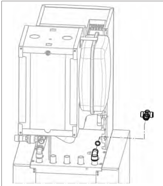
38. Kreuzstück (Pos. 6.5) mit Überwurfmutter-Seite und Flachdichtung (Pos. 6.20) an den zuvor montierten Anschlussbogen am RL Speicher montieren.
