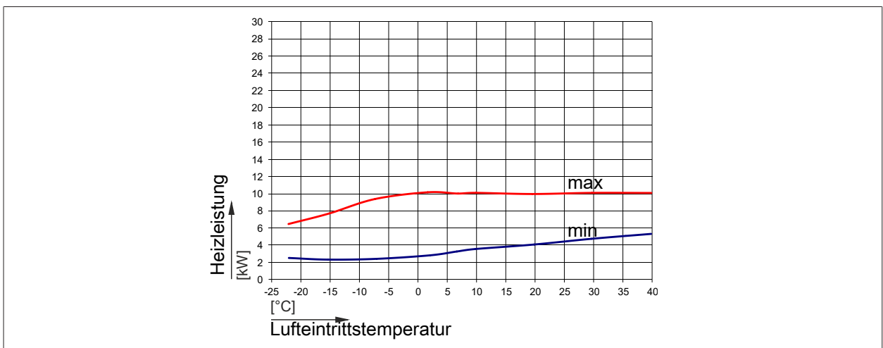
Abb. 6: Heizleistung CHA-10 bei einem Vorlauf von 45 °C
