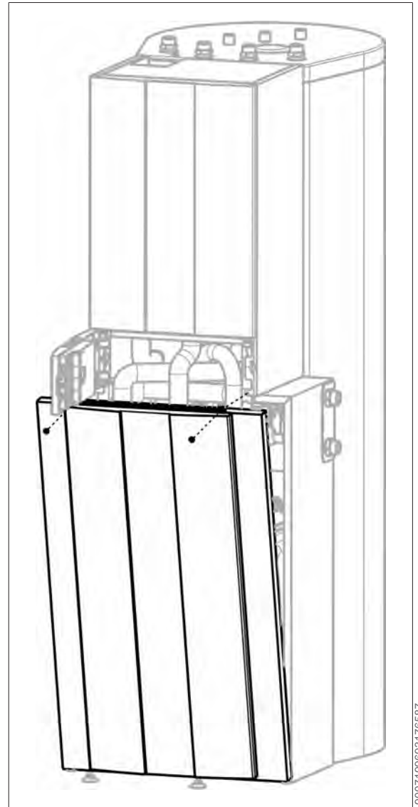
54. Frontblech mit Schrauben (Pos. 13.5) montieren.
