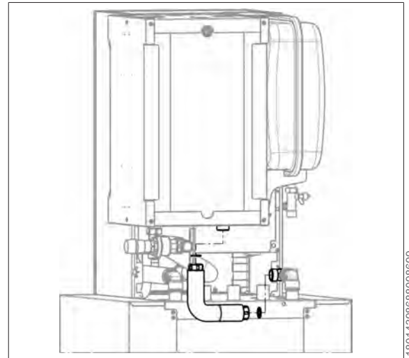
40. Wellrohr Anbindung Puffer (Pos. 6.11) mit 2x Flachdichtungen (Pos. 6.20) seitlich am Kreuzstück und am Pufferspeicher verschrauben.
