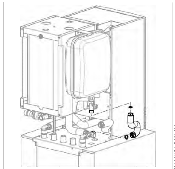
41. Wellrohr DN 15 (Pos. 6.13) gemäß Bild vorbeugen und unter Verwendung der Flachdichtungen (Pos. 6.19 und 6.20) mit Kreuzstück und Ausdehnungsgefäß verbinden.
