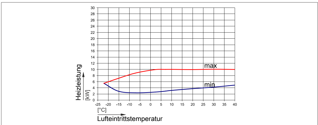
Abb. 7: Heizleistung CHA-10 bei einem Vorlauf von 55 °C
