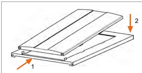
53. Frontverkleidung Hydraulik (Pos. 14.1) in Frontblech (Pos. 14.2) montieren.
