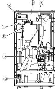
SEITENSICHT
