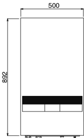
FRONTANSICHT
