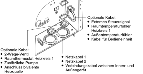
Führung der optionalen Kabel und Netzkabel (Ansicht ohne interne Verdrahtung)
