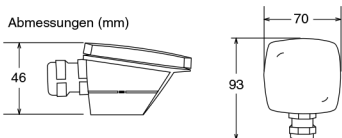
Abmessungen (mm)
