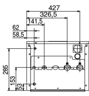
ANSICHT VON UNTEN
