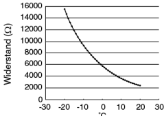
Kennlinie des Speichertemperaturfühlers
