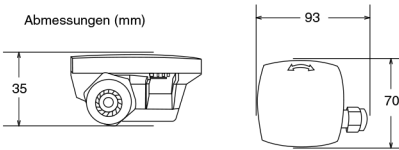
Abmessungen (mm)
