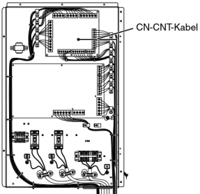
Mit optionaler Platine
