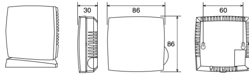
Abmessungen (mm)
