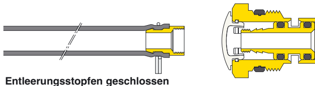
Entleerungsstoppfen geschlossen
