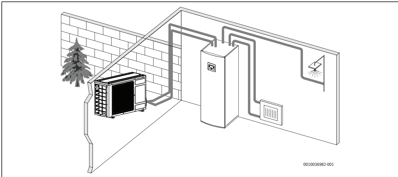
Bild 2 Wärmepumpe als Außeneinheit, Inneneinheit AWS M mit integriertem Warmwasserspeicher und elektrischem Zuheizter
