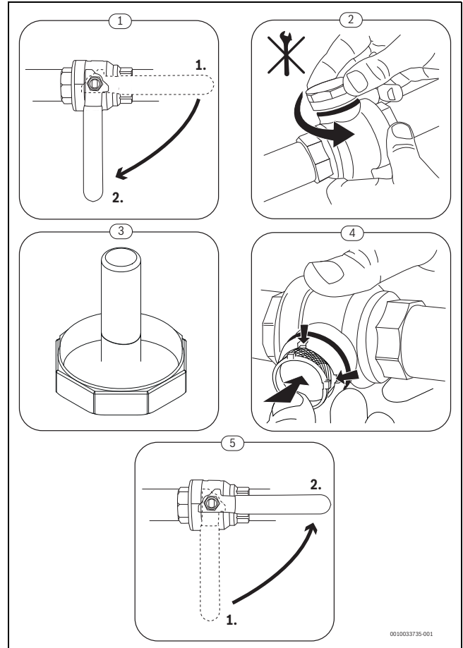
Bild 40 Siebreinigung
