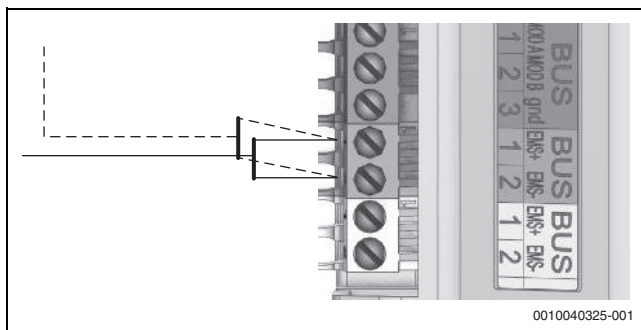
Bild 22 EMS-Anschluss
