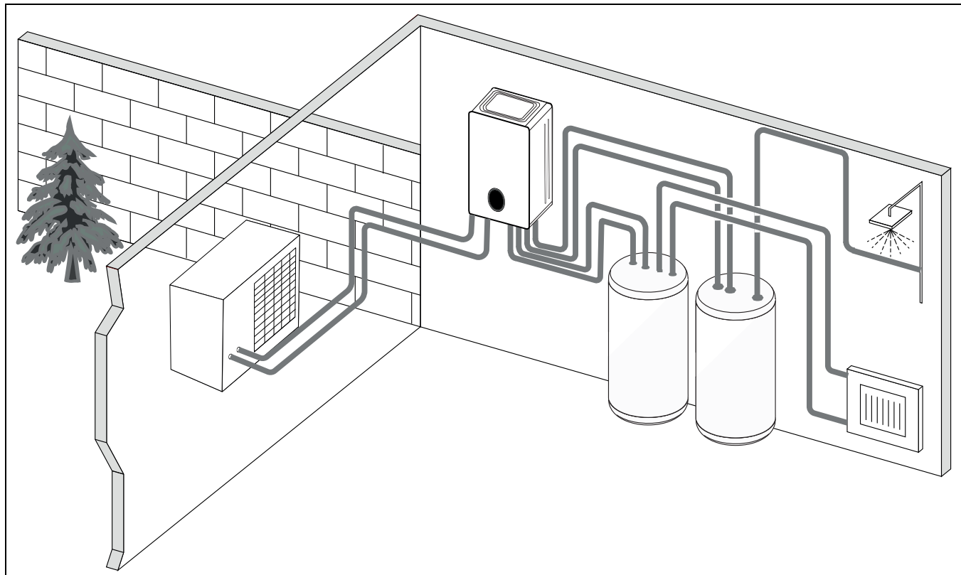
Bild 7 Wärmepumpe AW OR, Inneneinheit Compress 5800/6800i 12 E mit elektrischem Zuheizung und externem Warmwasserspeicher
