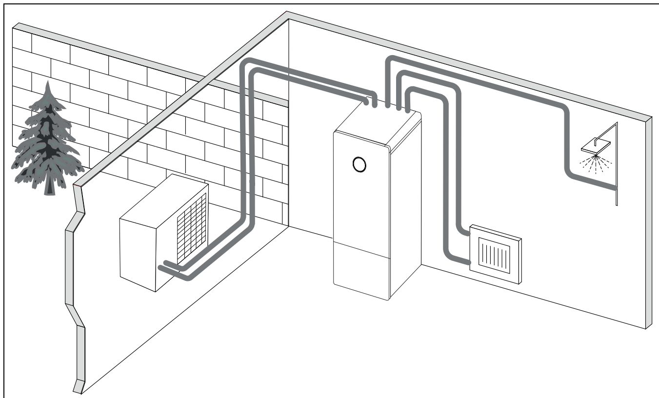
Bild 7 Wärmepumpe AW OR, Inneneinheit Compress 5800/6800i 12 M mit integriertem Warmwasserspeicher und elektrischem Zuheizung
