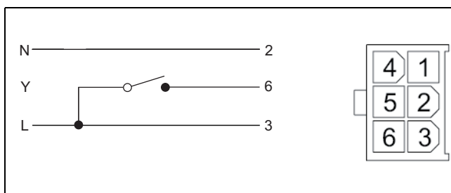
Bild 21 Molex-Stecker
