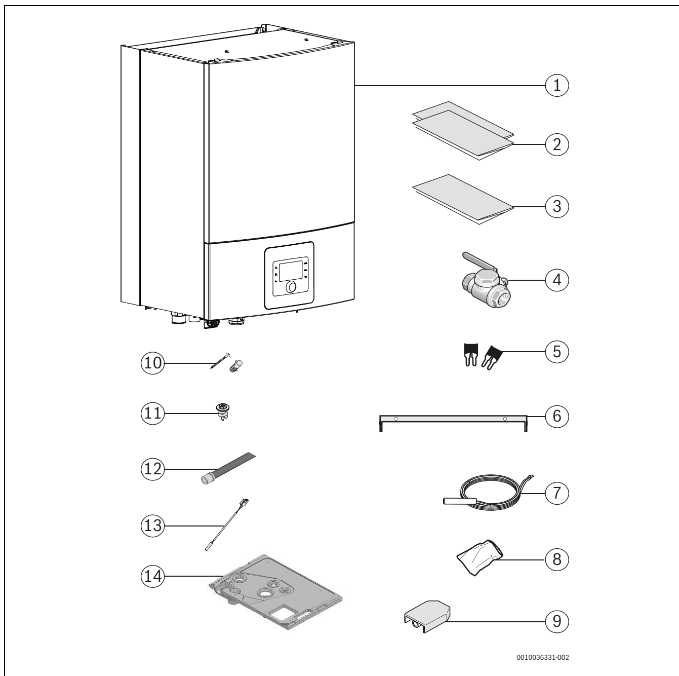
Bild 2 Lieferumfang
