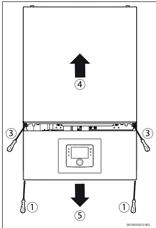
Bild 6 Frontverkleidung abnehmen
