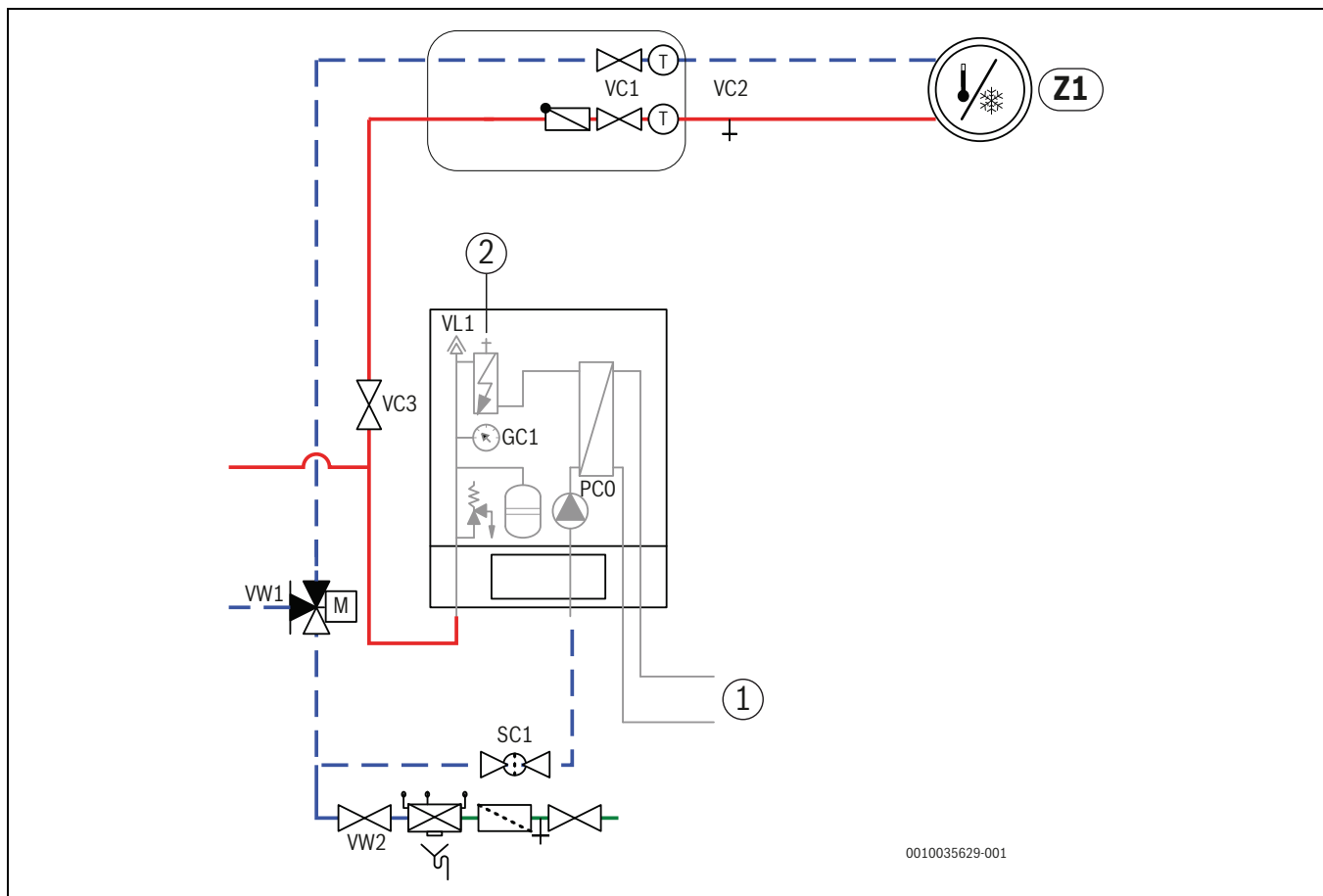
Bild 16 Inneneinheit mit integriertem elektrischem Zuheizgerät und Heizungsanlage
