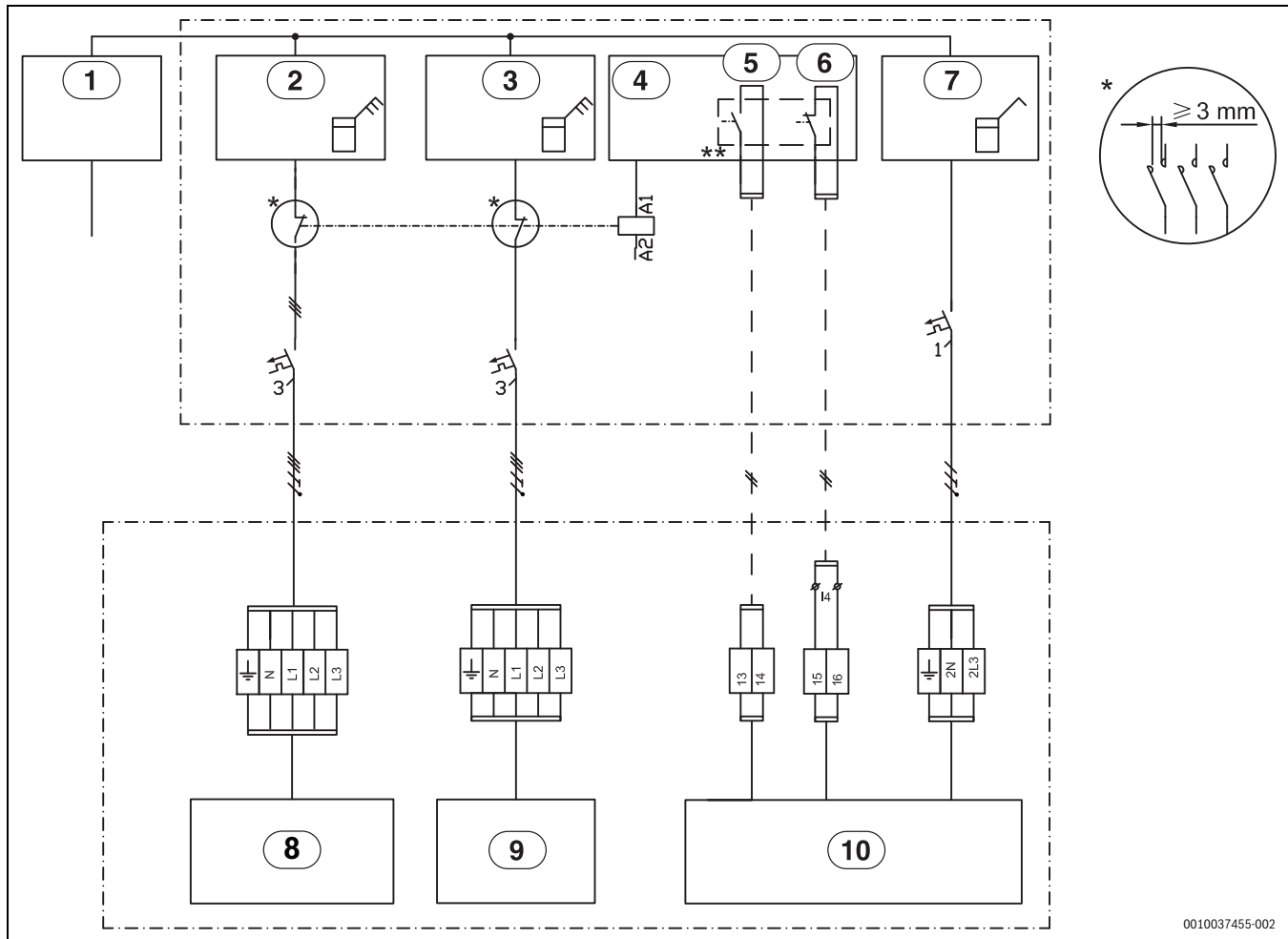
Bild 50 EVU Typ 1
