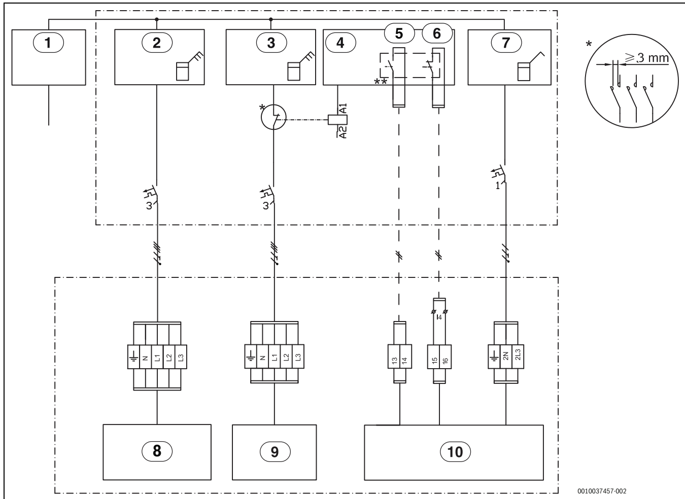
Bild 52 EVU Typ 3
