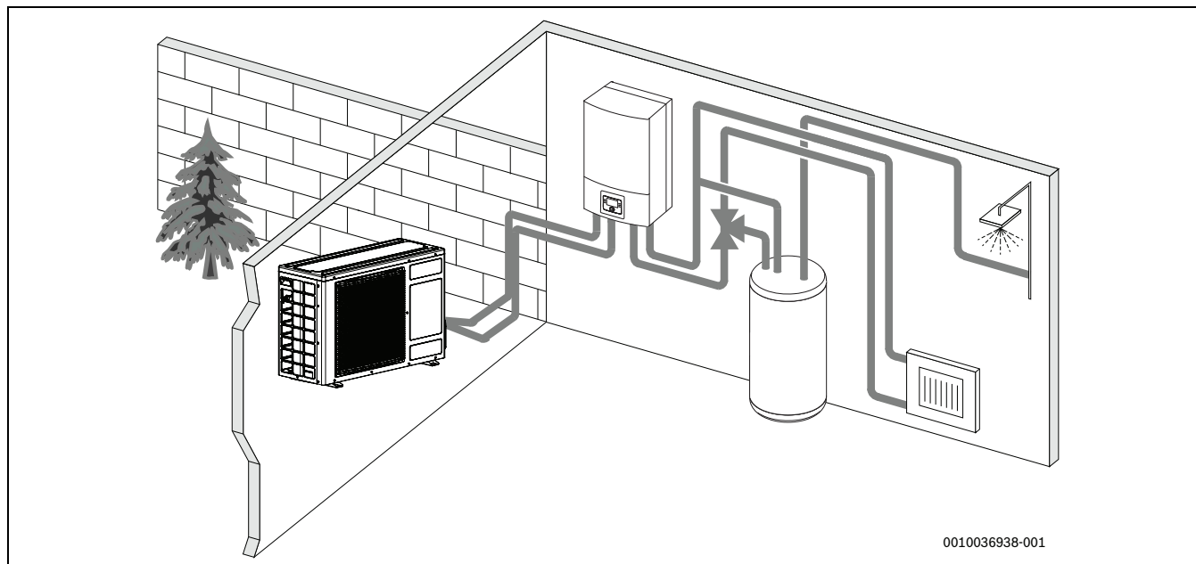
Bild 2 Wärmepumpe als Außeneinheit, Inneneinheit AWS E mit integriertem Warmwasserspeicher und elektrischem Zuheizung
