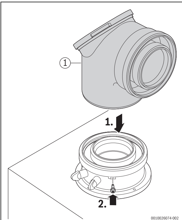
Bild 83 Abgaszubehör einsetzen und mit Schraube sichern
