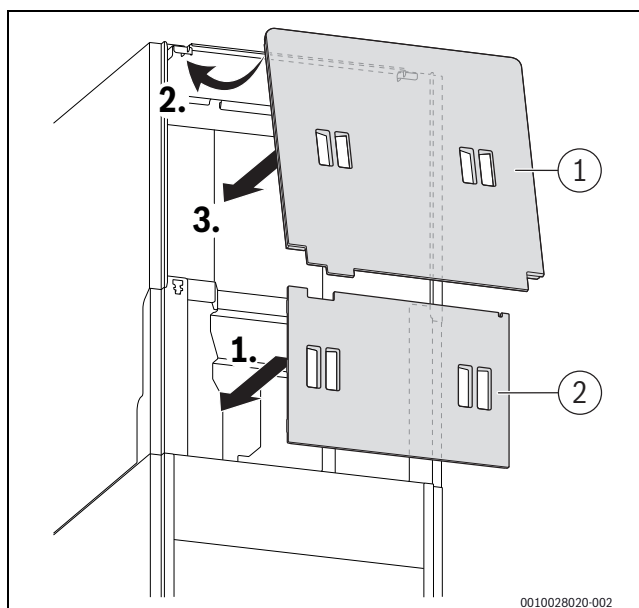
Bild 106 Wärmedämmung an der Rückseite anbringen (Zubehör SF 13)
