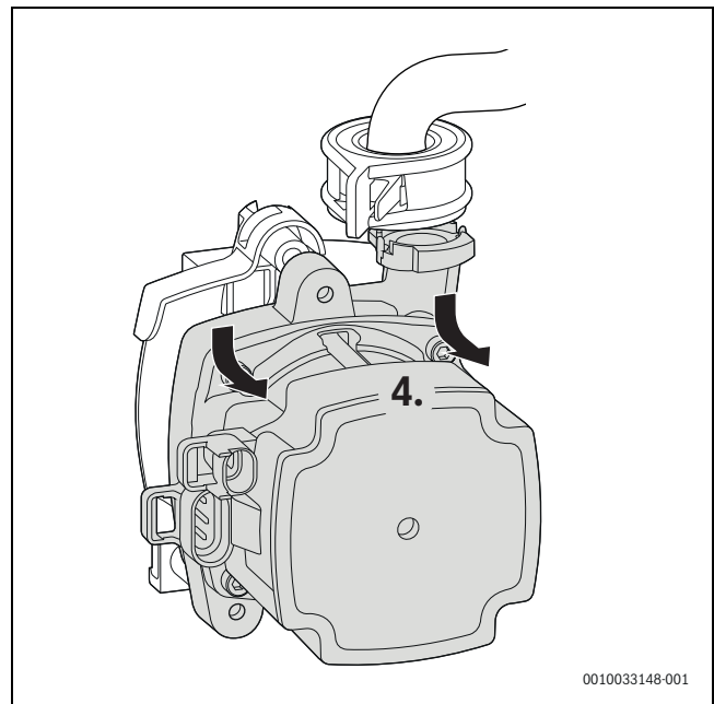
Bild 147 Heizungspumpe abnehmen
