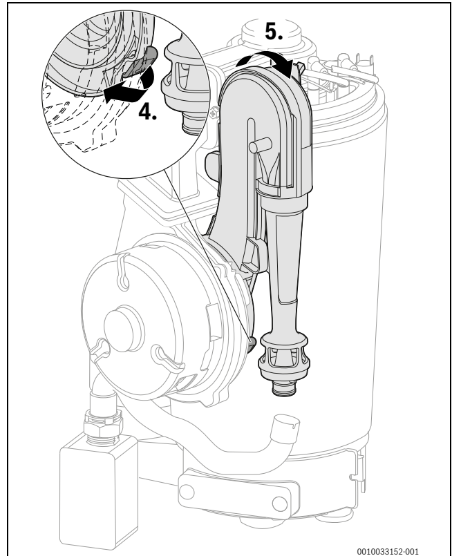
Bild 129 Venturirohr abnehmen
