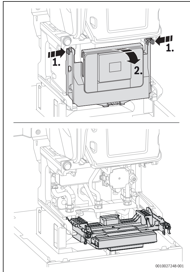
Bild 125 Steuergerät herunterklappen
