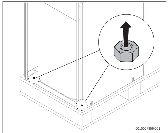
Bild 53 Transportsicherung unten an der Rückseite des Speichers entfernen
