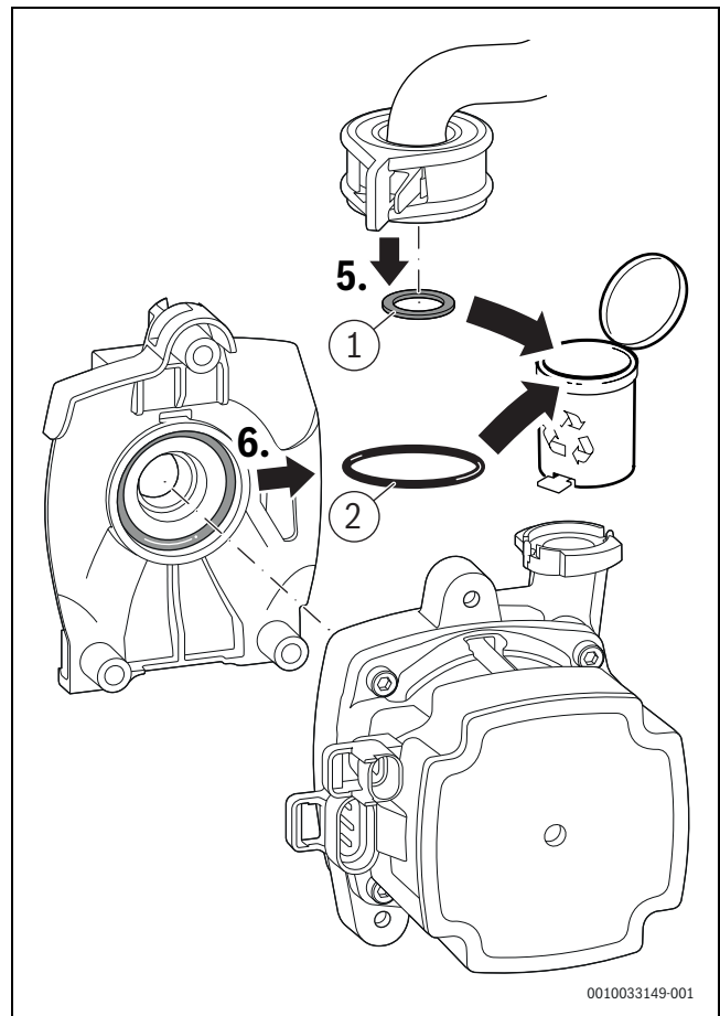
Bild 148 Dichtungen entsorgen
