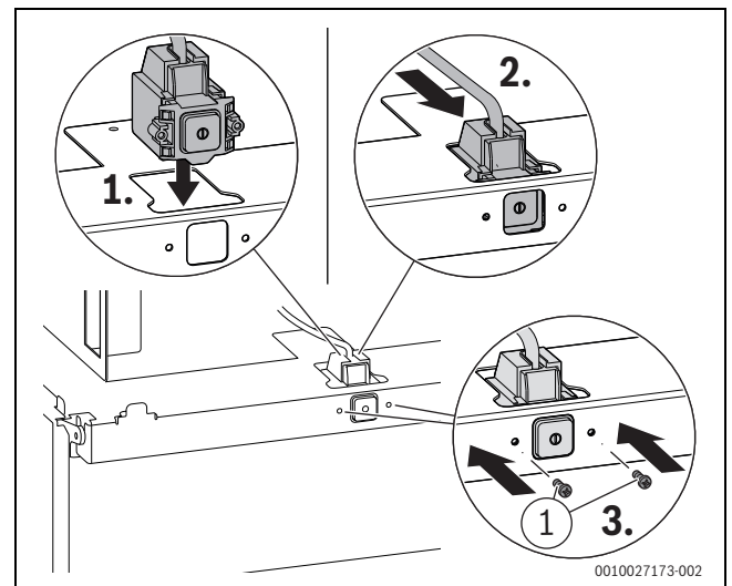
Bild 90 Schalter Ein/Aus befestigen
