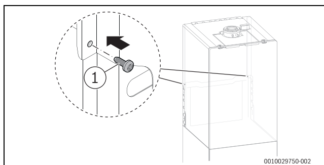
Bild 105 Seitenteile der Geräteverkleidung auf der linken und rechten Seite festschrauben
