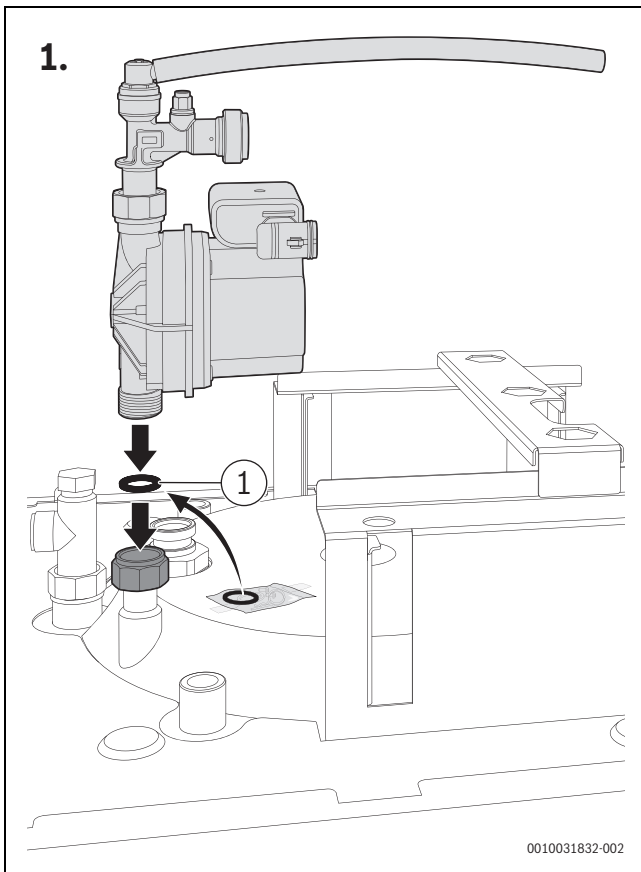
Bild 55 Schichtladepumpe einsetzen
