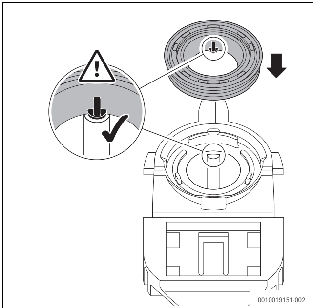
Bild 159 Neue Dichtung am Kondensatsiphon ausrichten
