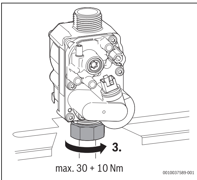
Bild 154 Anzugsdrehmoment beachten
