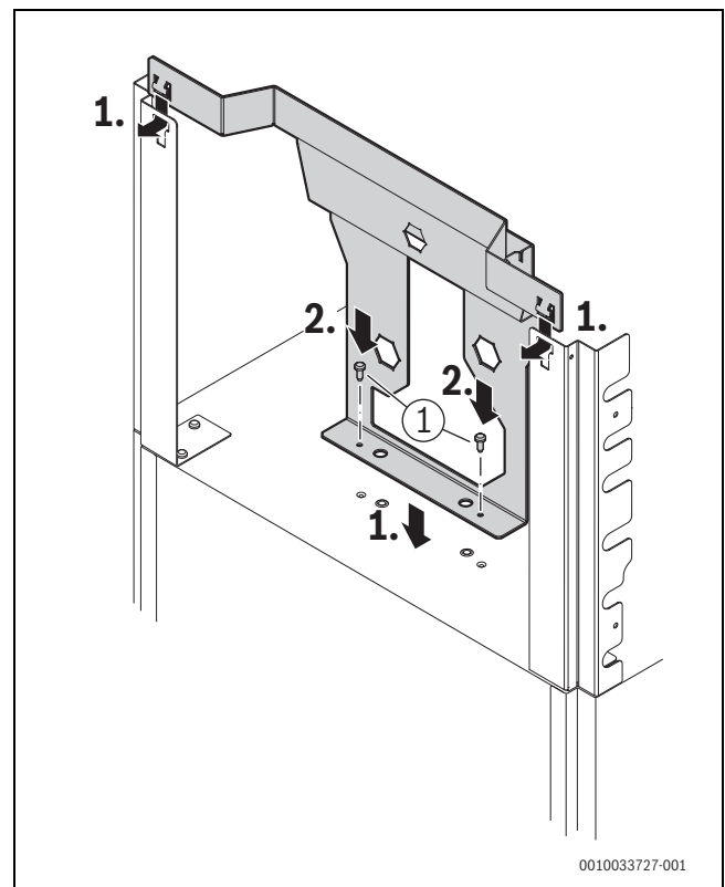
Bild 58 Basismodul (Zubehör CS 35) montieren – Schritt 2
