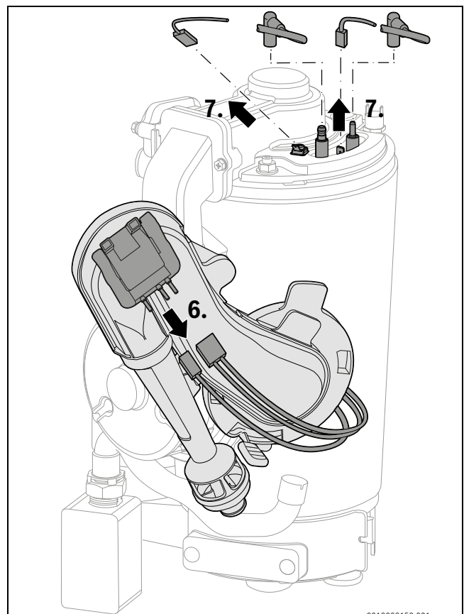
Bild 130 Kabel abziehen
