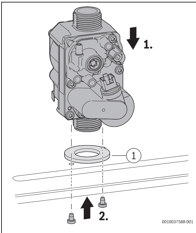
Bild 153 Gasarmatur einbauen
