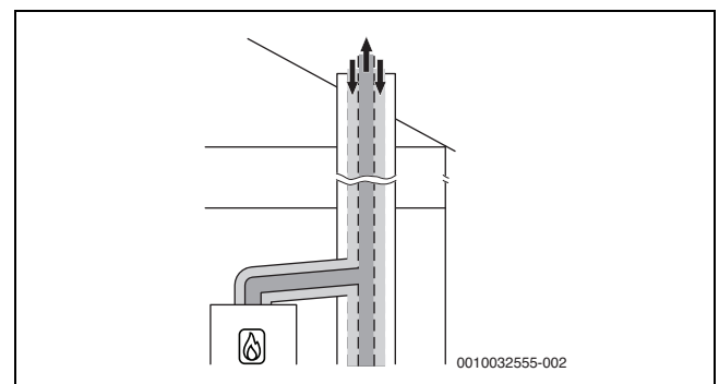
Bild 31 Konzentrische Luft-Abgas-Führung nach C 43x im Aufstellraum
