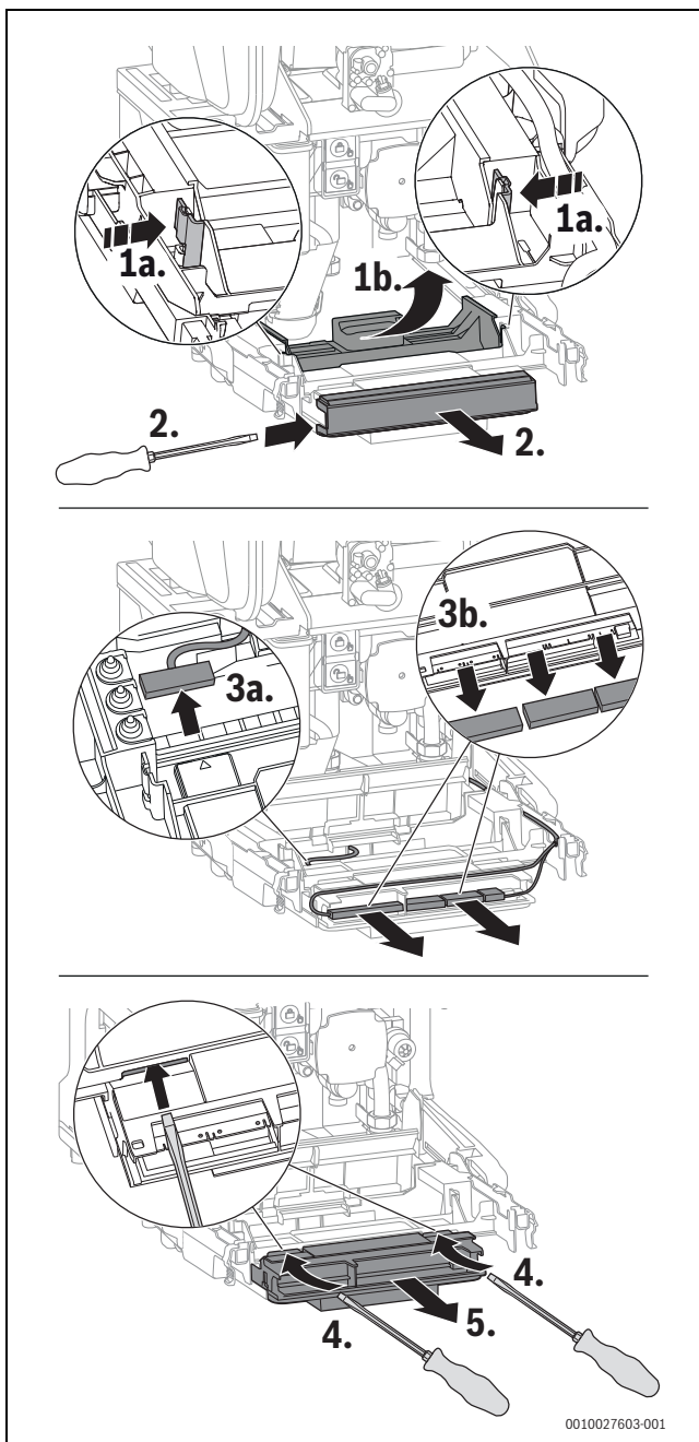
Bild 157 Steuergerät herausnehmen
