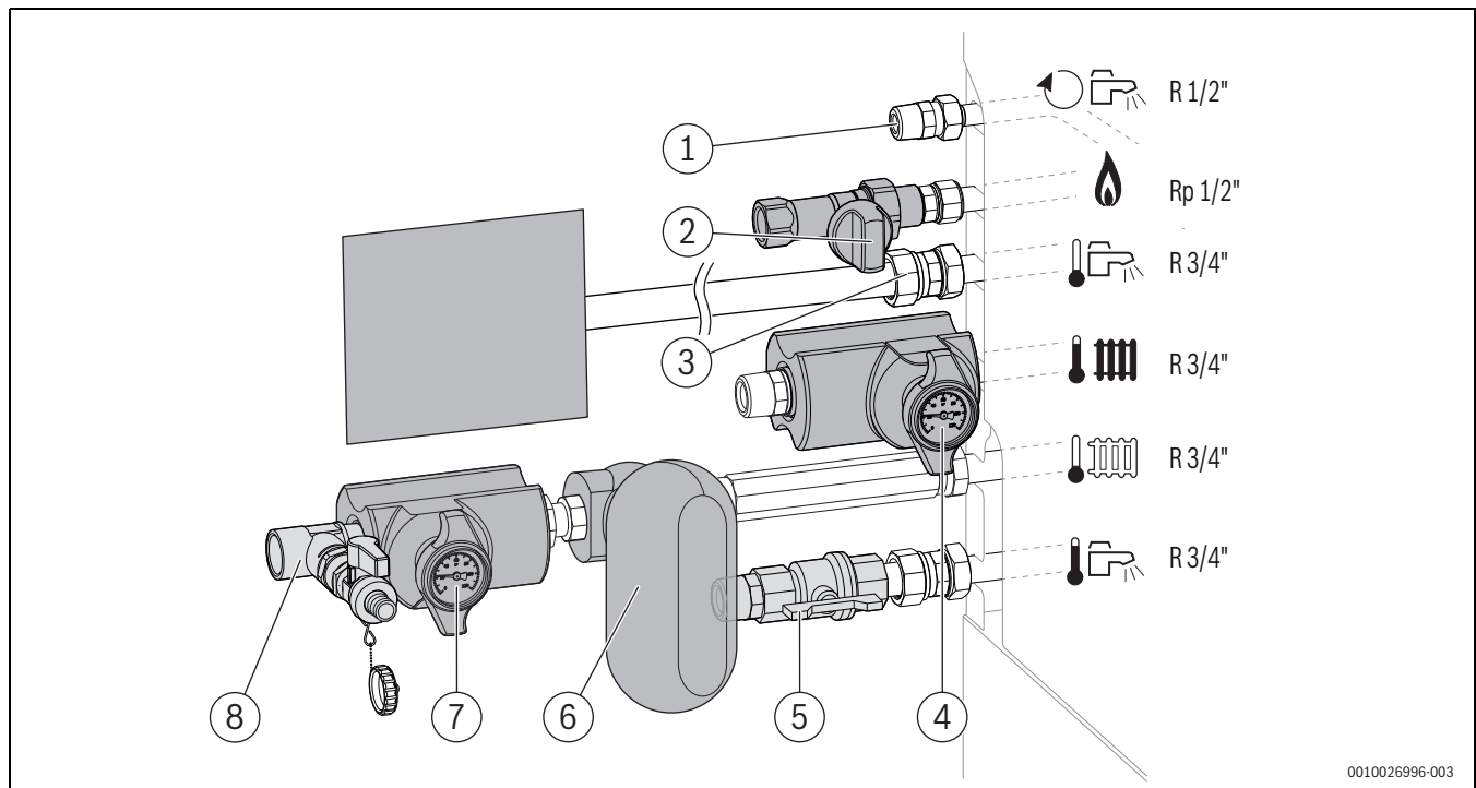
Bild 86 Armaturen-Set Zubehör CS 28-1 – Beispiel: Anschlüsse horizontal auf der linken Seite
