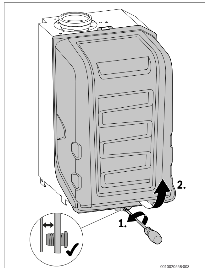
Bild 87 Brennerhaube abnehmen
