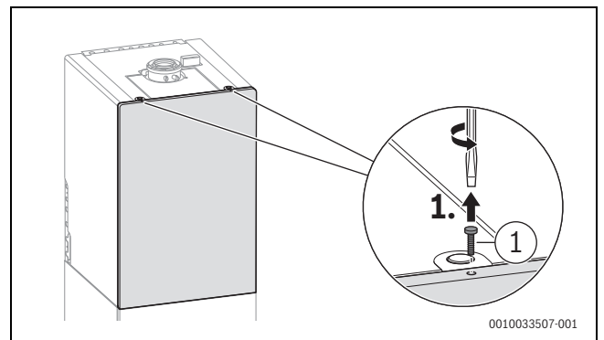
Bild 122 Sicherungsschraube lösen
