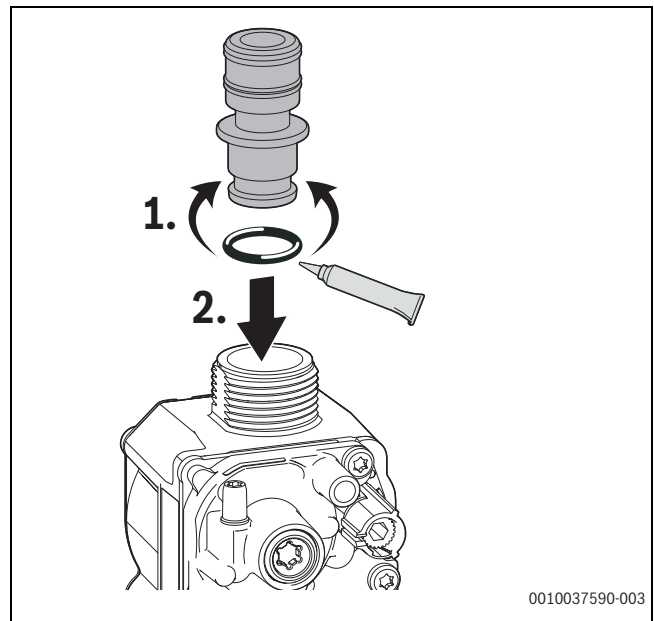
Bild 155 Gasdüse einsetzen
