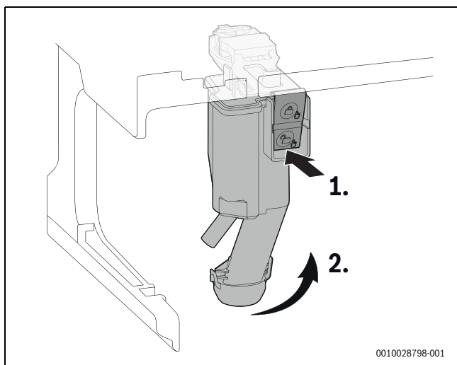
Bild 70 Kondensatsiphon herausnehmen
