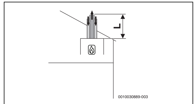
Bild 30 Vertikale konzentrische Luft-Abgas-Führung nach C 33x
