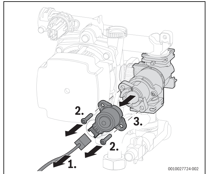
Bild 163 Motor am 3-Wege-Ventil ausbauen
