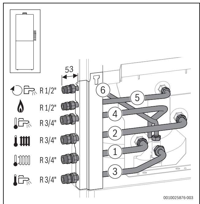
Bild 13 Ansicht von der Rückseite (Maß in mm): Zubehör CS 10 auf der rechten Seite montiert
