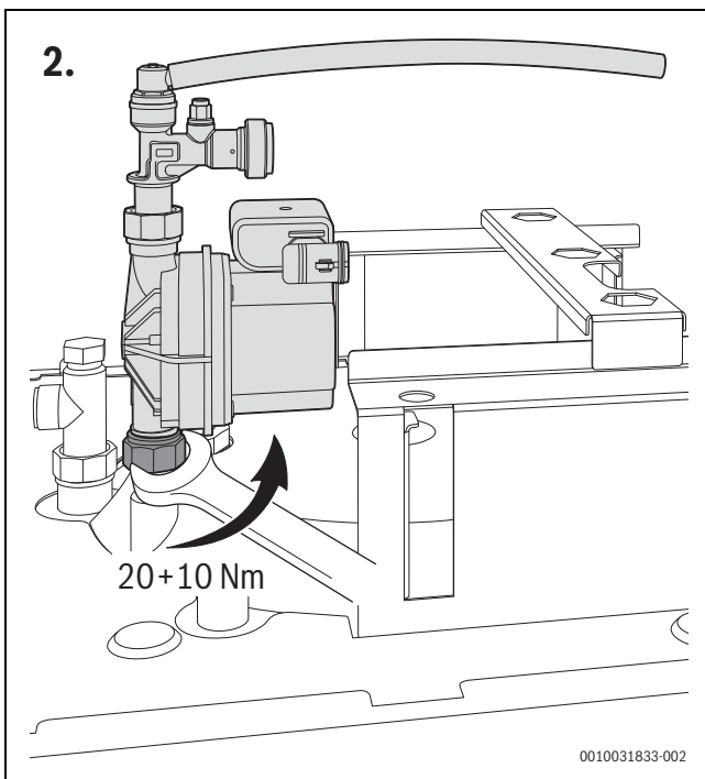
Bild 56 Anzugsdrehmoment beachten
