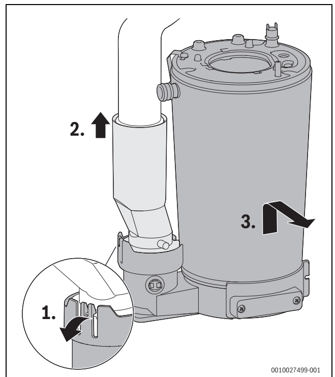
Bild 144 Wärmeblock ausbauen
