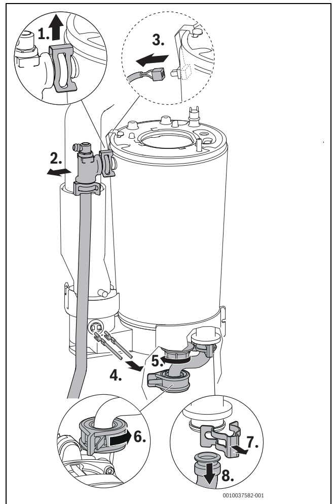
Bild 143 Vorlaufrohr lösen, Kabel abziehen und Rücklaufrohr lösen
