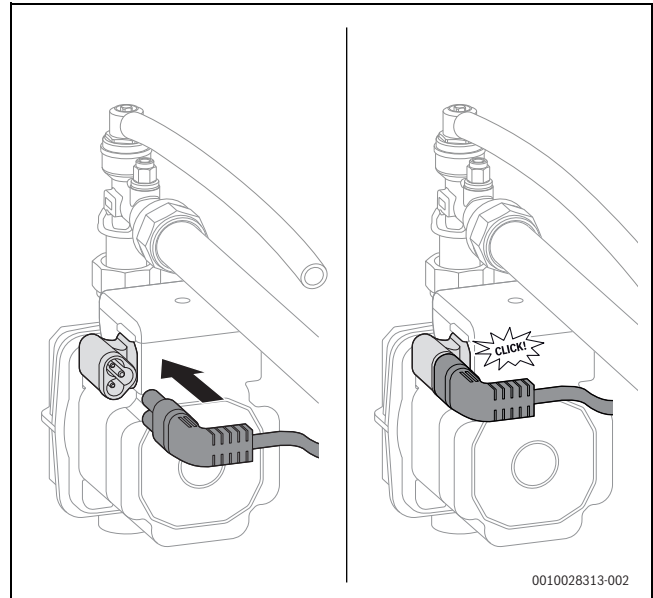
Bild 98 Schichtladepumpe elektrisch anschließen
