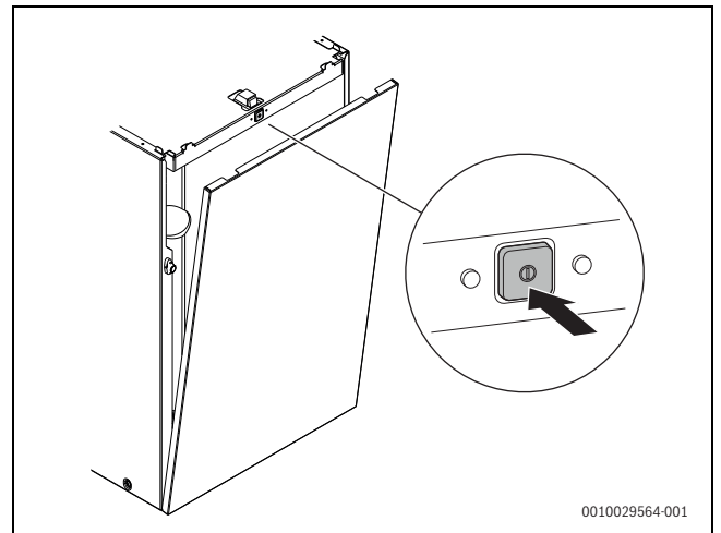
Bild 121 Gerät am Schalter Ein/Aus einschalten
