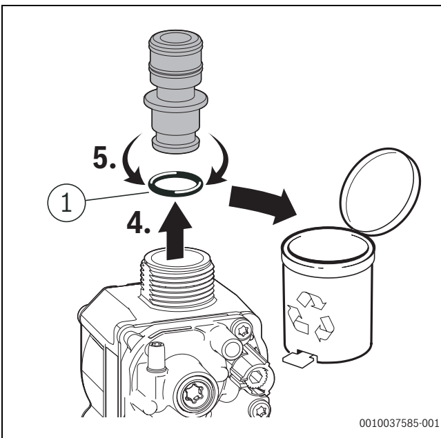
Bild 150 Gasdüse abnehmen
