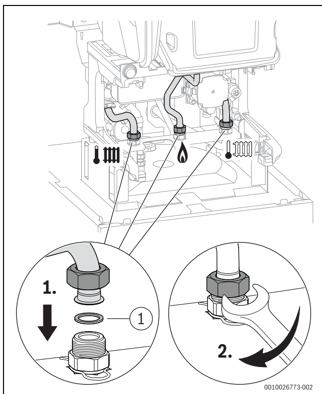
Bild 71 Heizungsvorlauf, Gas, Heizungsrücklauf anschließen
