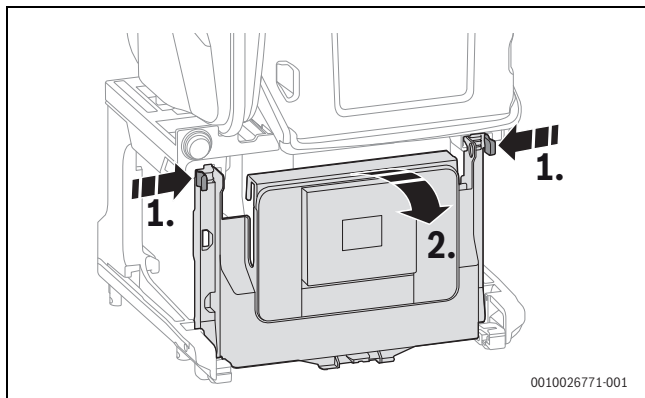
Bild 69 Steuergerät herunterklappen
