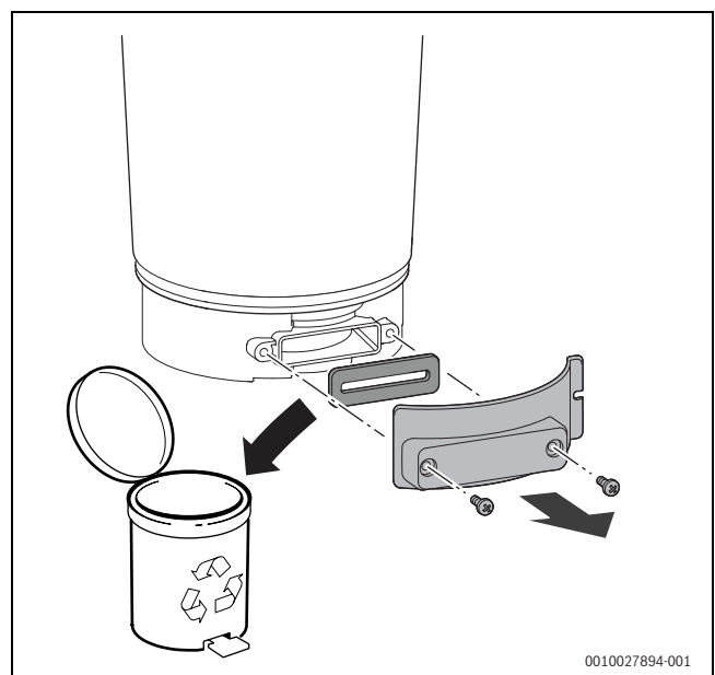
Bild 140 Prüföffnung öffnen
