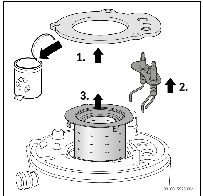
Bild 134 Brenner herausnehmen
