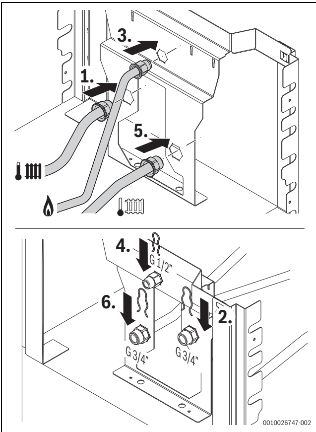
Bild 59 Heizungsanlass, Gasrohr und Heizungsanlass hinten einsetzen (Zubehör CS 35)
