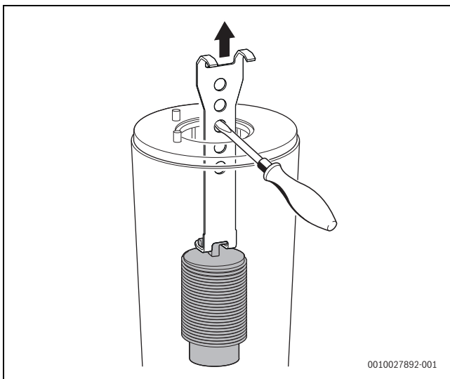
Bild 136 Unteren Verdrängungskörper herausnehmen
