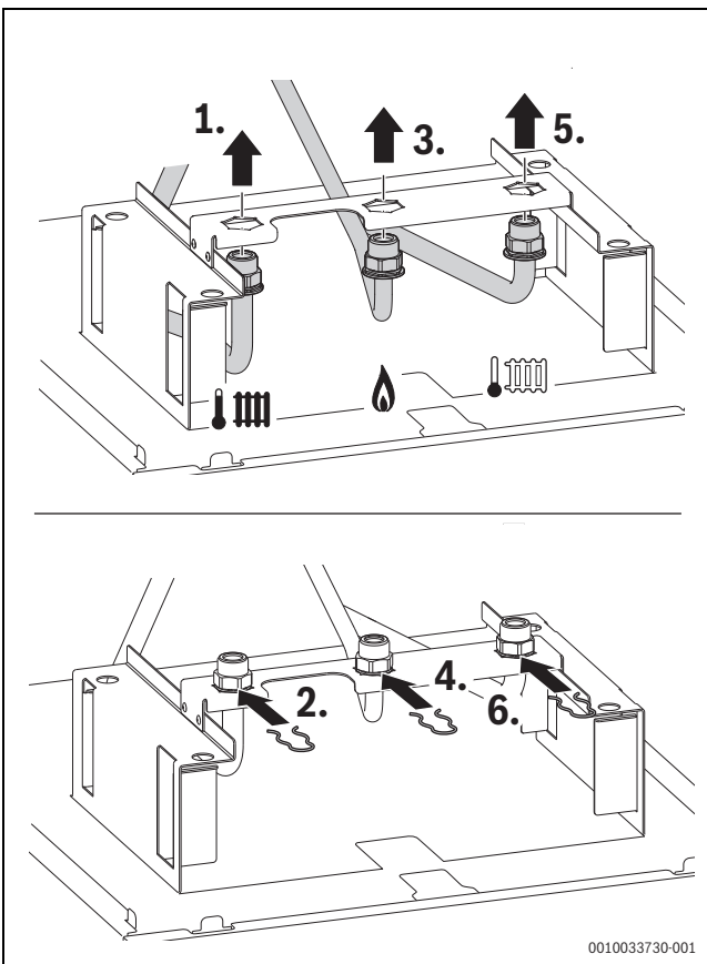
Bild 60 Heizungsanlass, Gasrohr und Heizungsanlass vorn einsetzen (Zubehör CS 35)
