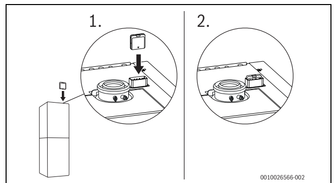
Bild 84 Control Key in den Key-Halter einstecken
