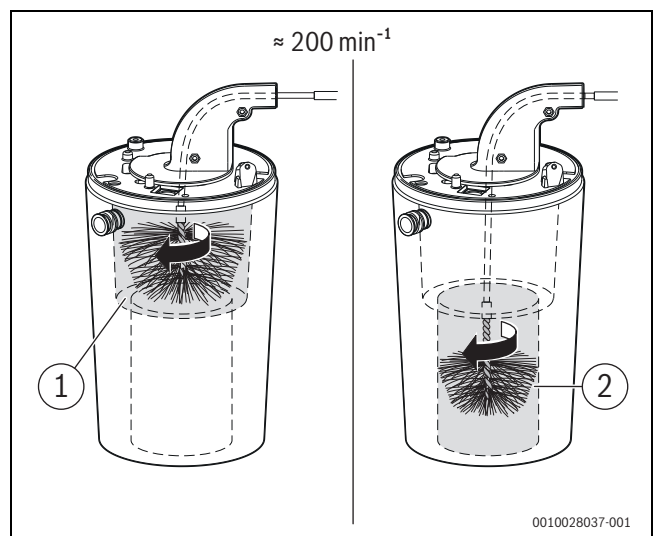
Bild 139 Wärmeblock reinigen (ca. 200 \text{ min}^{-1} , nur Rechtslauf)
