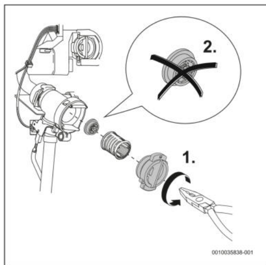
Bild 57 Durchflussbegrenzer entfernen.
