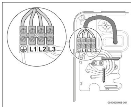
Bild 43 Anschluss oben
