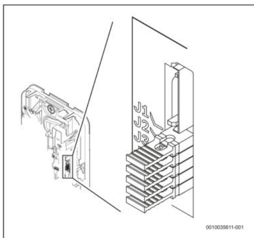
Bild 39 Mitgelieferte elektronische Brücken
