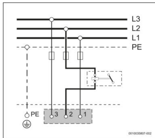
Bild 42 Schaltplan
