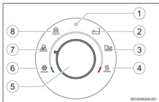
Bild 5 Bedienfeld
