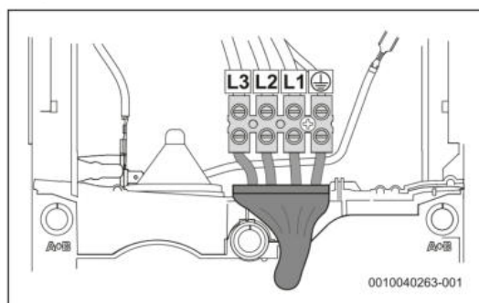
Bild 52 Anschluss unten kurze Kabel
