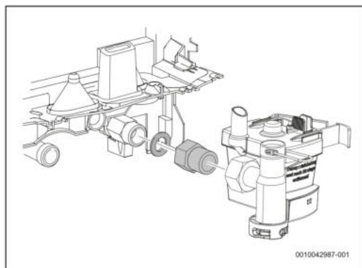
Bild 29 Zusätzliche Buchse
