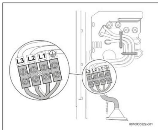
Bild 44 Anschluss unten
