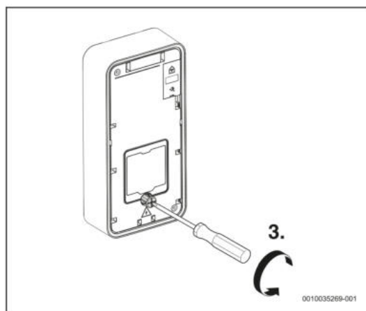
Bild 11 Schraube lösen
