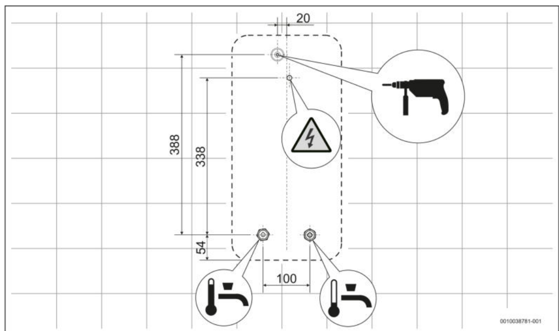
Bild 3 Abmessungen in mm
