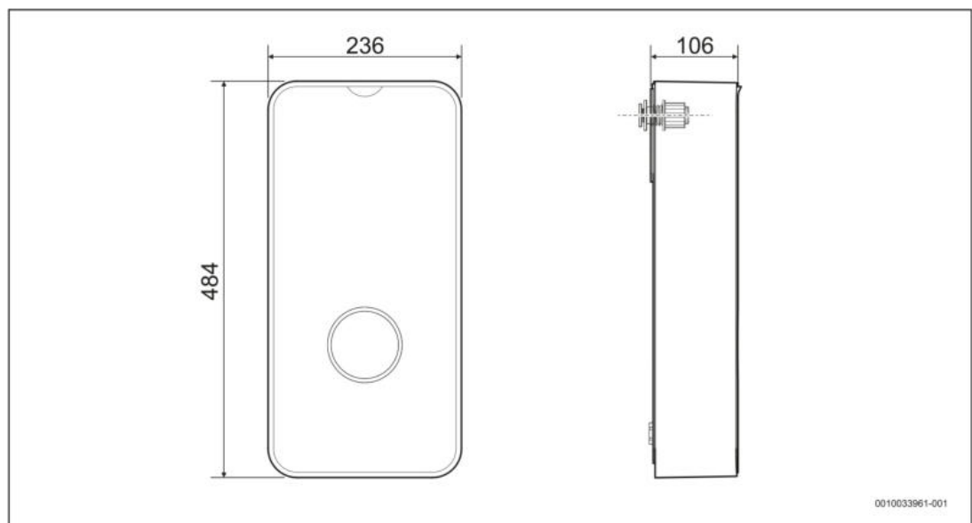
Bild 2 Abmessungen in mm
