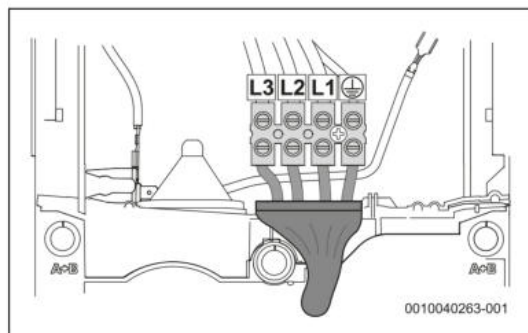
Bild 45 Anschluss unten für kurze Kabel
